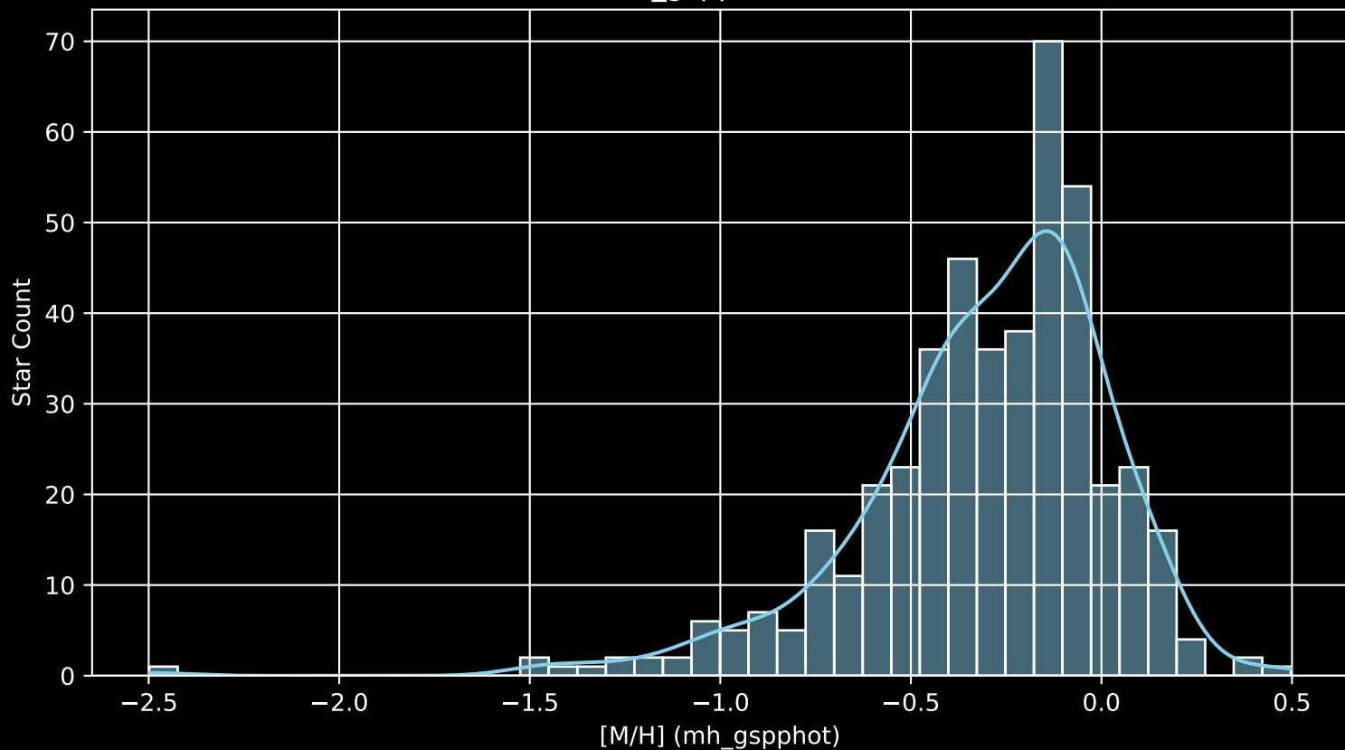
GALAH DR4 Field: [6602] [M/H] (mh_gspphot) (n= 452)
