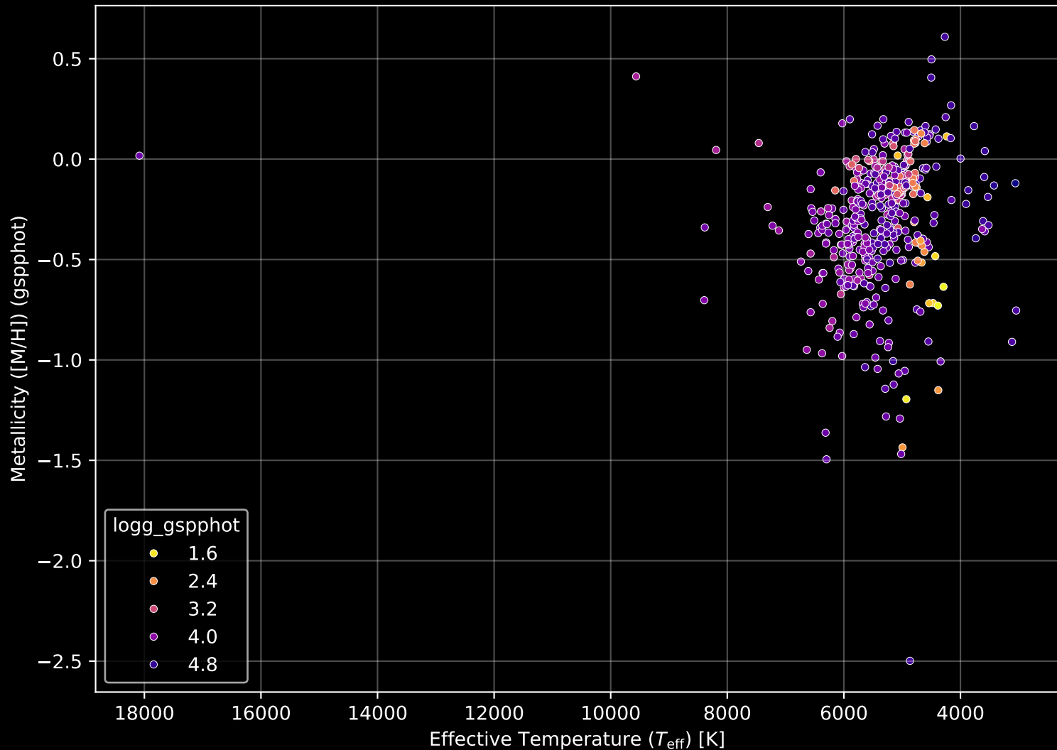
GALAH DR4 Field: [6602] Stellar Population Parameters (n= 453)
